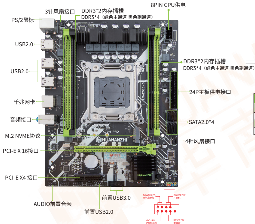
图1-1 X79M PRO主板图解
