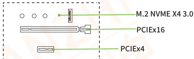
图2-4 PCI扩展插槽
